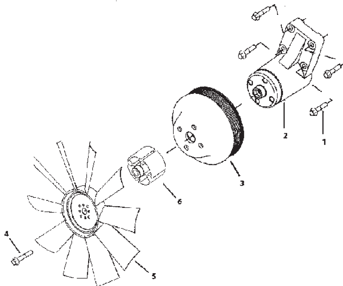
FAN AND FAN DRIVE
