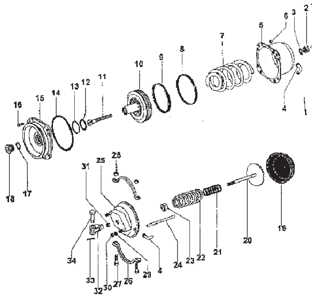
REAR BRAKE ACTUATOR (S-CAM)
